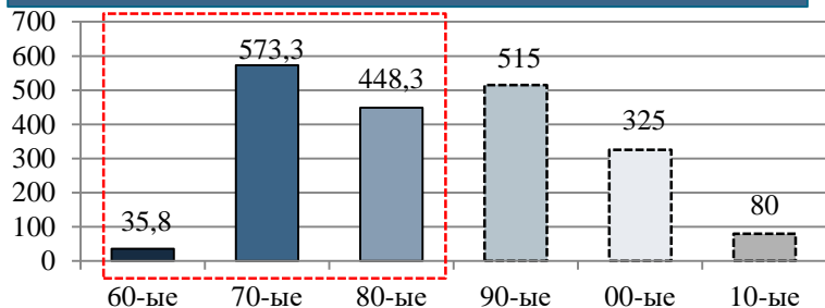
Анализ износа. Трансформаторы 35-110 кВ (МВА)
